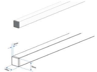
END CAP
